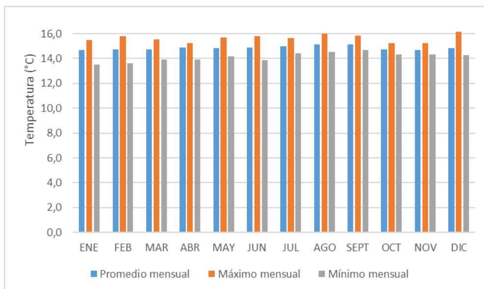
Figura 13.5. Temperatura media mensual (2020-2024), Estación REMMAQ Carapungo
